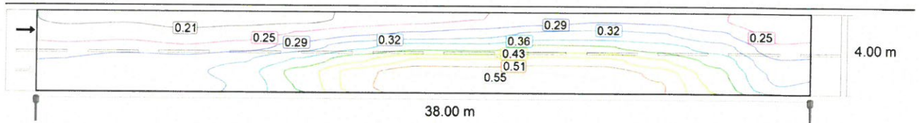
Observator 2: Valoarea de întreținere, densitatea luminii cu carosabil uscat [cd/m²] (Linii Isolux)
