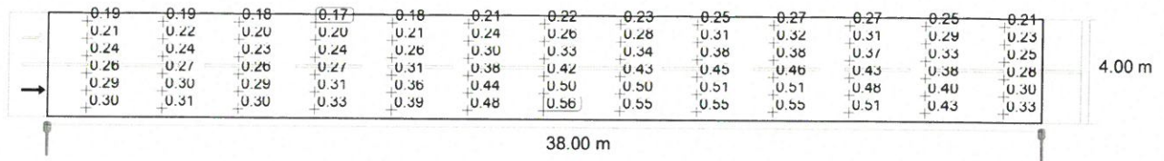
Observator 1: Valoarea de întreținere, densitatea luminii cu carosabil uscat [cd/m²] (Raster valoric)
